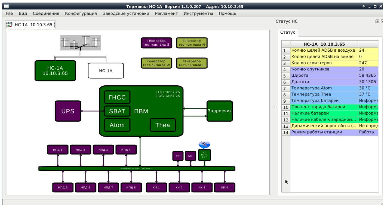
Рисунок 3 – Главное окно программы
