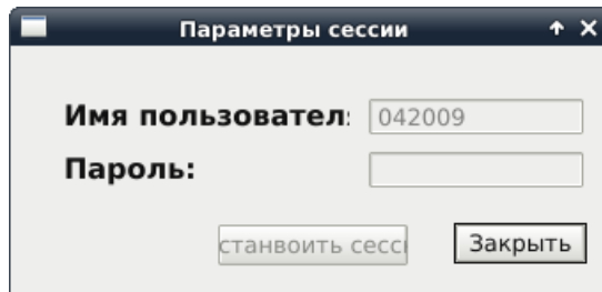
Рисунок 5 – Установить сессию
