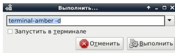
Рисунок 2 – Окно «Выполнить»
