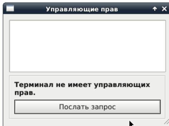
Рисунок 6 – Управляющие права
